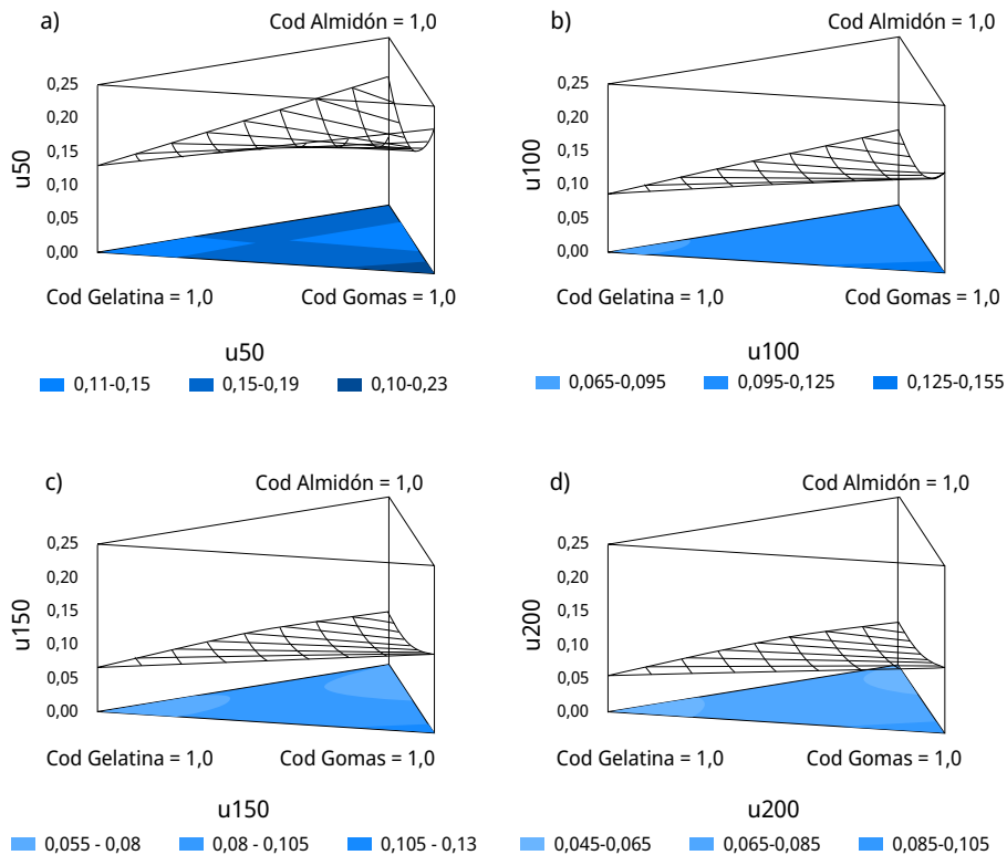
FIGURA 3. Gráficas de superficie de respuesta estimada para la viscosidad aparente de las bebidas lácteas a base de lactosuero, a diferentes gradientes de deformación a) 50 \text{ s}^{-1} , b) 100 \text{ s}^{-1} , c) 150 \text{ s}^{-1} y d) 200 \text{ s}^{-1} , en función de la concentración de almidón, gelatina y mezcla de gomas guar y garrofín codificadas.
